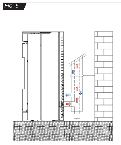
FIG. 5 Sortie fumées arrière concentrique. Modèle: GLOBO 6 kW, GLOBO 8 kW, GLOBO 10 kW
