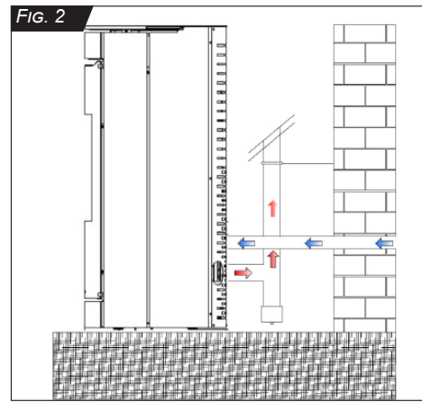
FIG. 2 Sortie fumées arrière et prélèvement de l'air comburant directement de l'extérieur au travers d'un tube d'arrivée de l'air comburant. Modèle: GLOBO 6 kW, GLOBO 8 kW, GLOBO 10 kW
