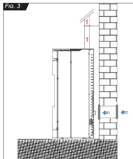
FIG. 3 Sortie fumée supérieure simple paroi et prélèvement de l'air comburant de l'extérieur au travers d'une ouverture dans le mur de la pièce. Modèle: GLOBO 6 kW UP, GLOBO 8 kW UP, GLOBO 10 kW UP
