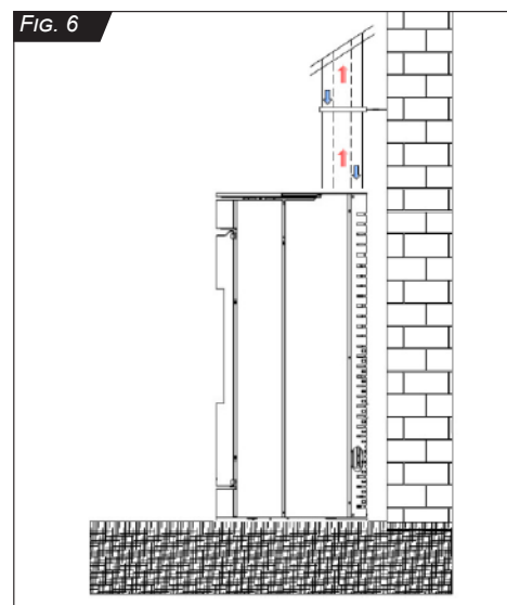
FIG. 6 Sortie fumées supérieure concentrique. Modèle : GLOBO 6 kW UP/C, GLOBO 8 kW UP/C, GLOBO 10 kW UP/C
