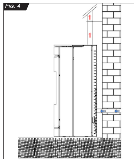
FIG. 4 Sortie fumées supérieure simple paroi et prélèvement de l'air comburant directement de l'extérieur au travers d'un tube d'arrivée de l'air comburant. Modèle: GLOBO 6 kW UP, GLOBO 8 kW UP, GLOBO 10 kW UP
